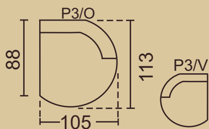
Divan end round right/left закругленный диван левый/правый
